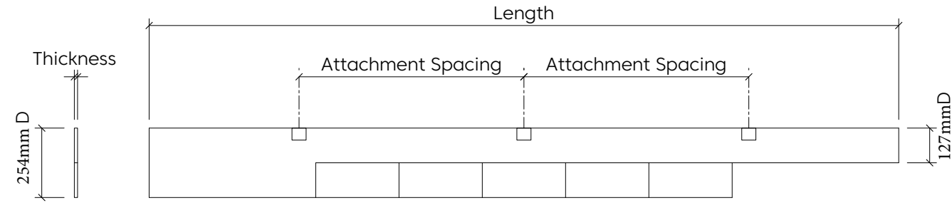
Elevation
